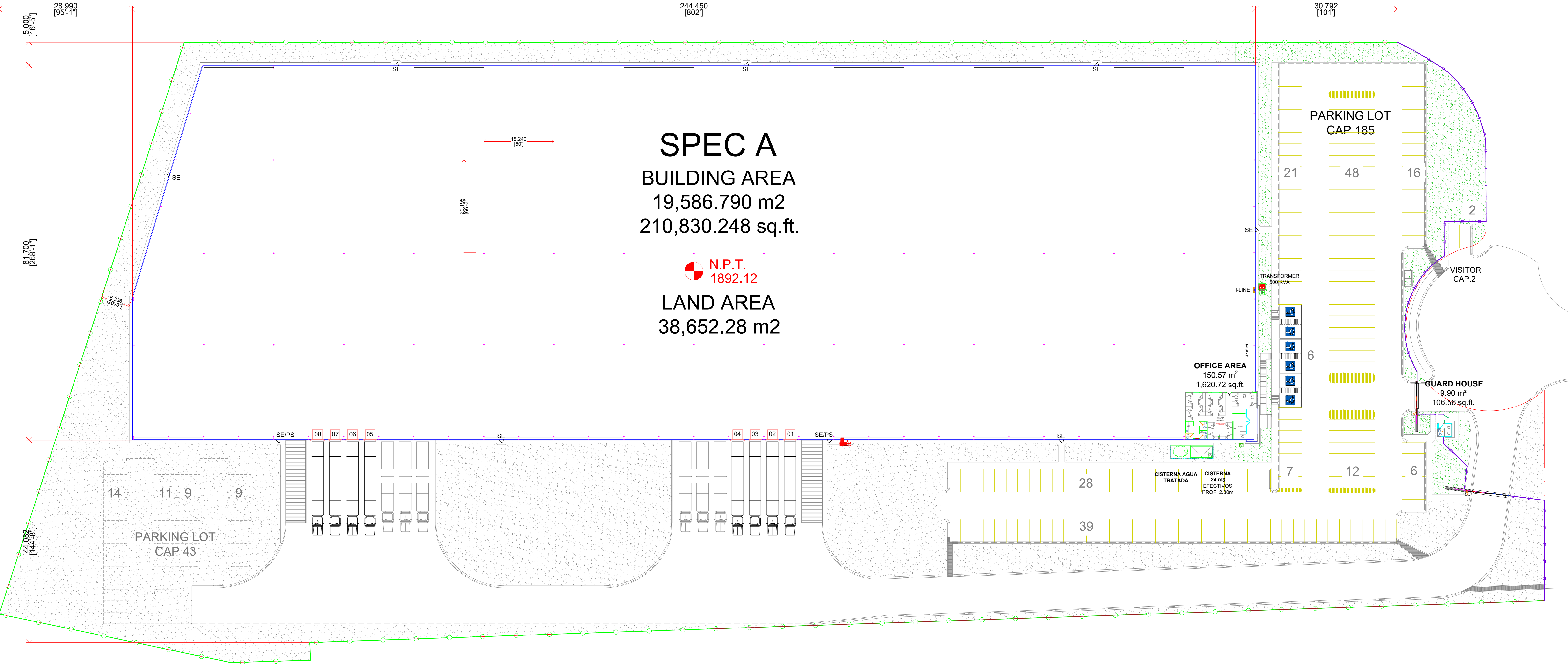
PLANTA ARQUITECTONICA ARCHITECTURAL LAYOUT
